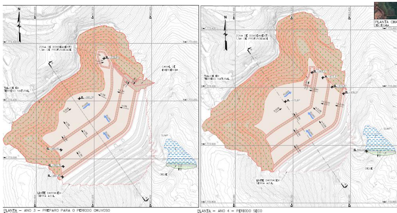
Figura 7: Projeto BVP – Descaracterização Elevação (chuvoso e seco – período).
