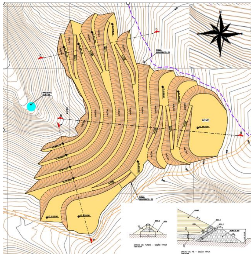
Figura 15: ECJ (Aço e Gnaiss - Mista) – AMDE.
