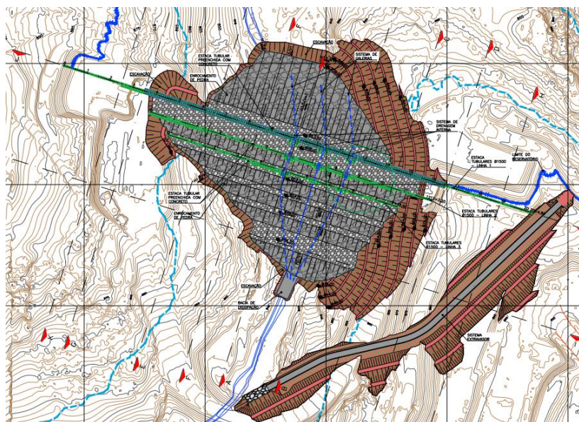
Figura 14: ECJ (Aço e Gnaiss - Mista) – Canal Extravassor / ECJ: Linha de tubos.
